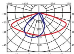
光束角70度-140度
