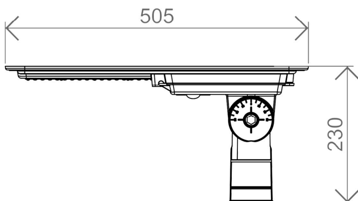
主视图
